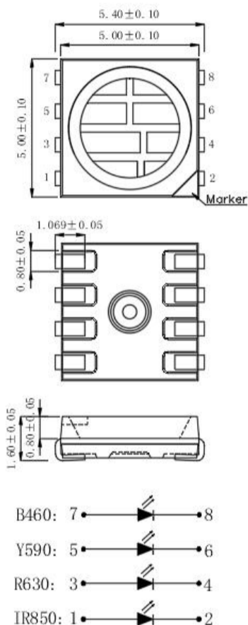
封装尺寸 Package Dimensions
