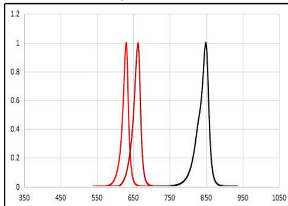
光谱特性图
