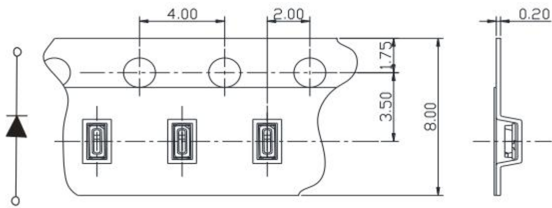
Reel Dimensions 卷轴尺寸
